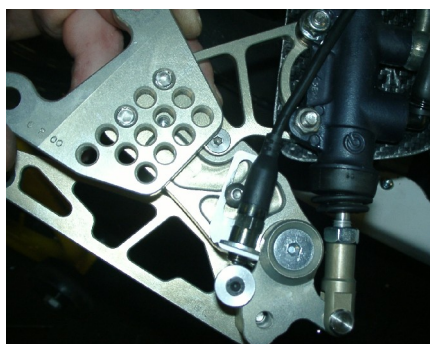
Vormontage Fußrastenanlage rechts Assembly footrest system on right side
