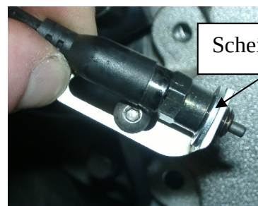
Montage Bremslichtschalter an Bremslichthalter Assembly Stopp light switch
