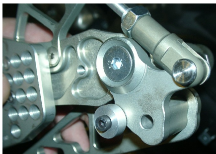
Befestigung Bremsbetätigungsstift Fastening break valve pin
