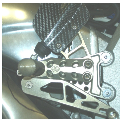
M8x30 DIN 7991
